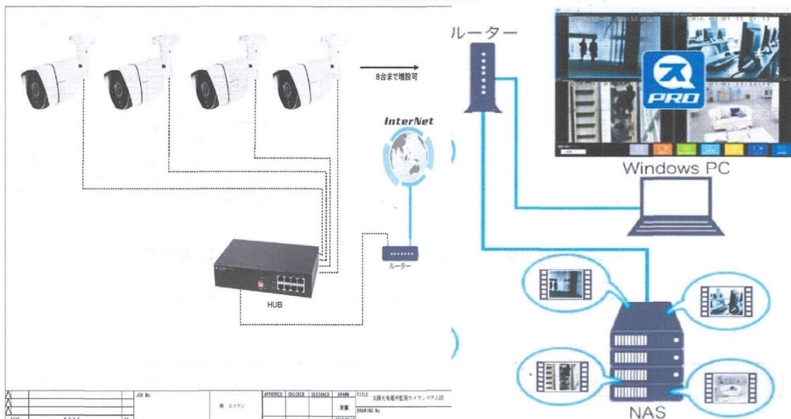
システム構成参考図
